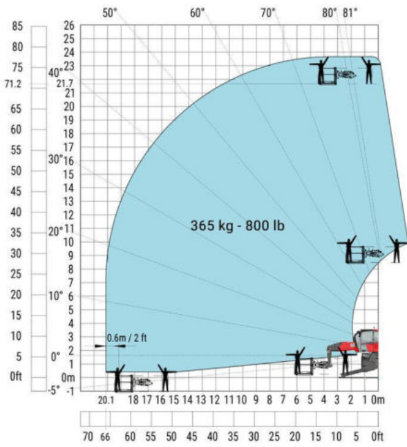
Drehung an abgesenkten Stützen mit 365 kg Arbeitskorb
