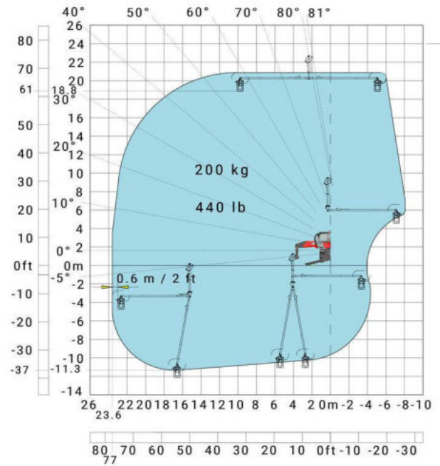
Drehung mit abgesenkten Stützen mit 3D negativ
