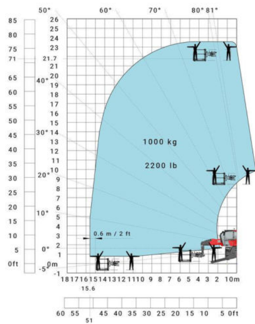
Drehung an abgesenkten Stützen mit 1000 kg Arbeitskorb
